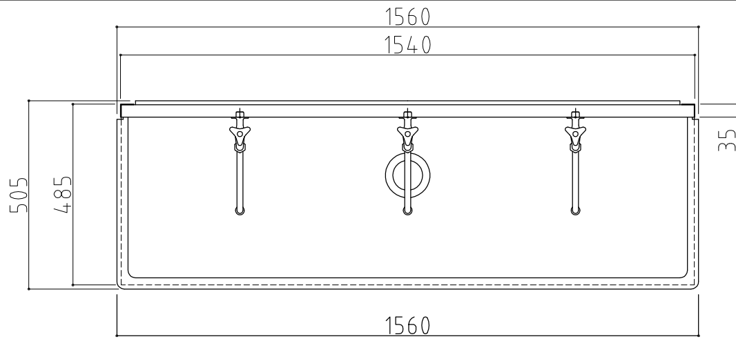
平面図
