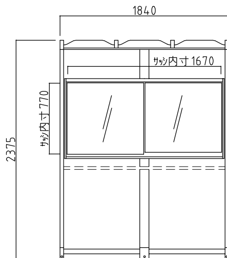
正面図
