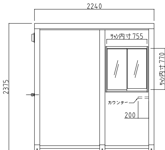
左側面図
