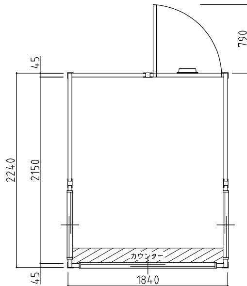
平面図
