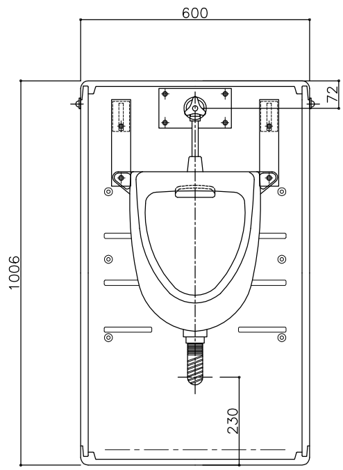
正面図 1
