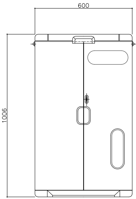
正面図 2
