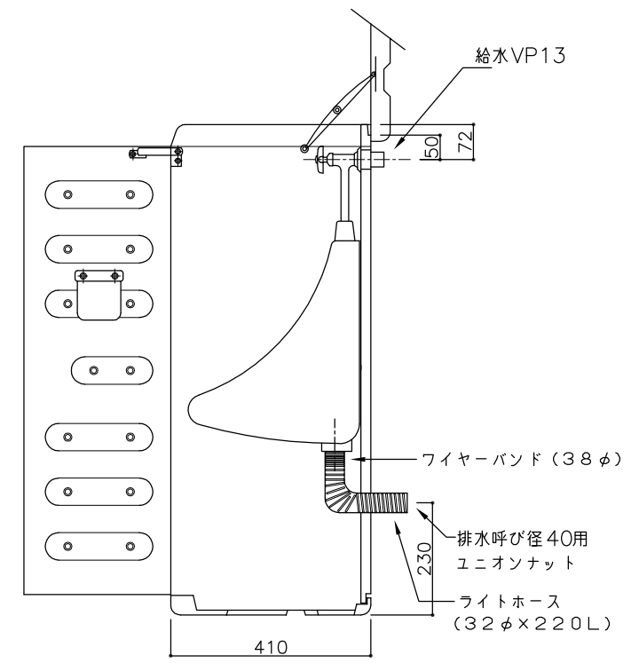
側面図
