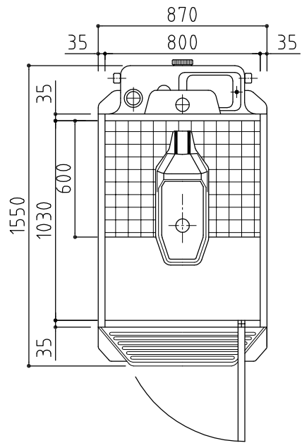
平面図
