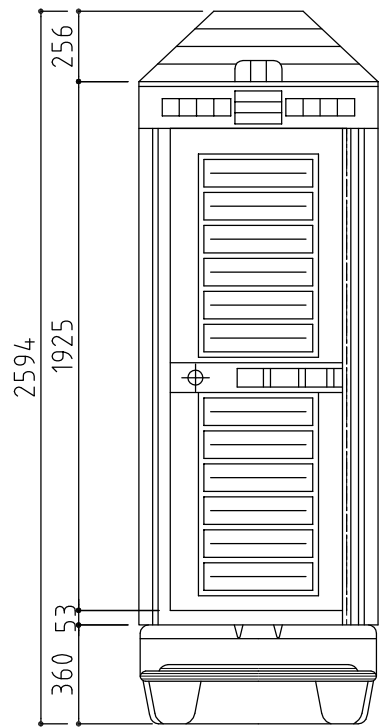
正面図
