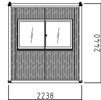
右側面図
