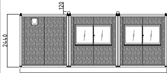
左側面図
