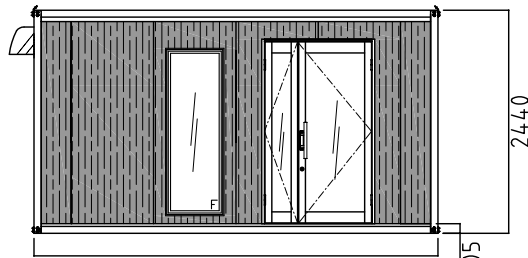
正面図
