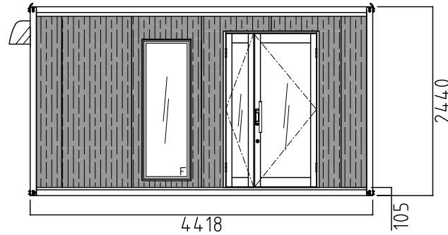
正面図
