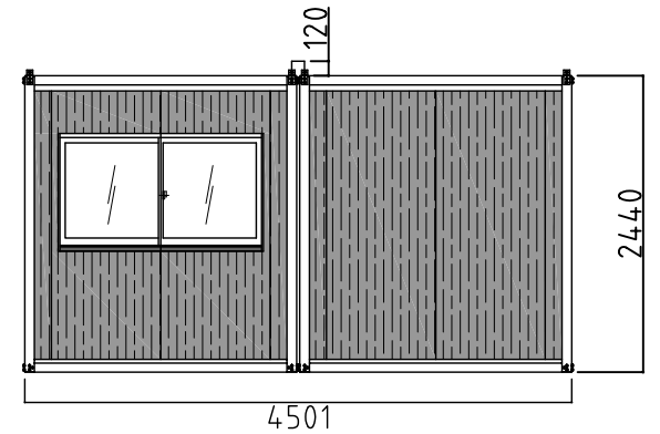
右側面図
