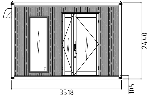
正面図
