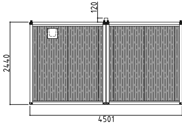
左側面図
