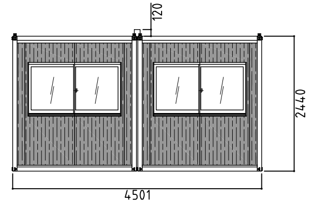
右側面図
