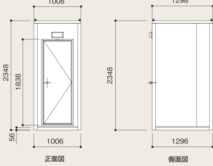
正面図
