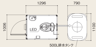
500L排水タンク
