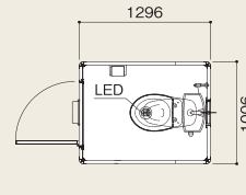
A-3型 水洗洋式 ラッピングパネル仕様
