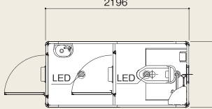
B-2型 水洗兼用式
