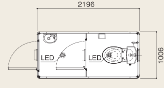
B-3型 水洗洋式 ラッピングパネル仕様
