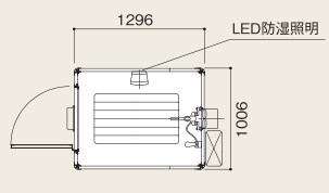
A-6型 シャトレ水洗 100V電気式洋式型
