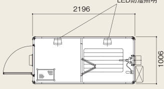
B-6型 浴室 電動換気扇 16号給湯器付
