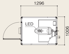
A-4型 シャワー室 電動換気扇 16号給湯器付
