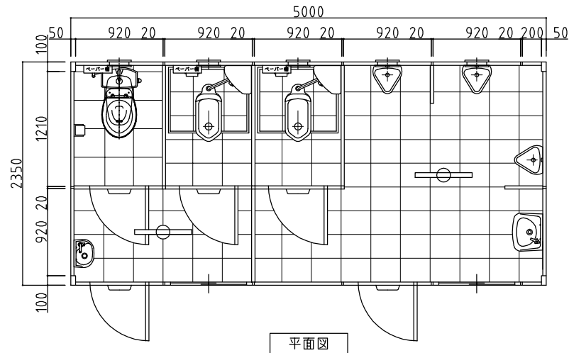
平面図
