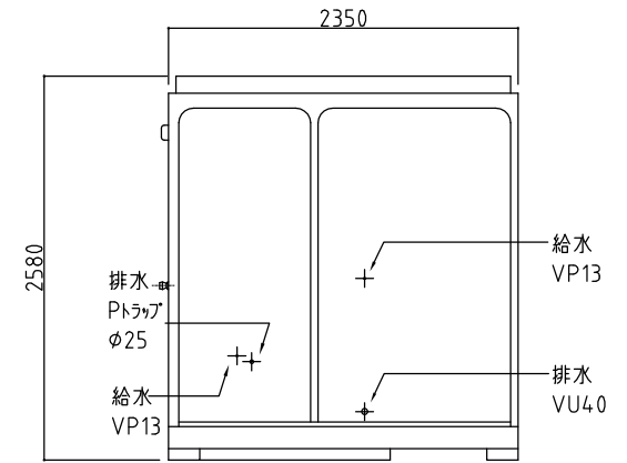
右側面図
