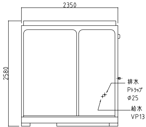
左側面図
