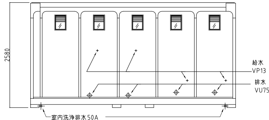
背面図
