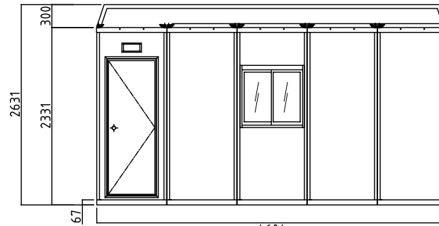
正面図
