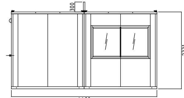
右側面図
