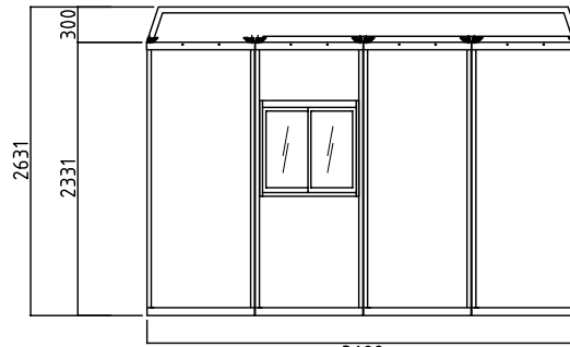
背面図
