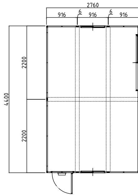
平面図
