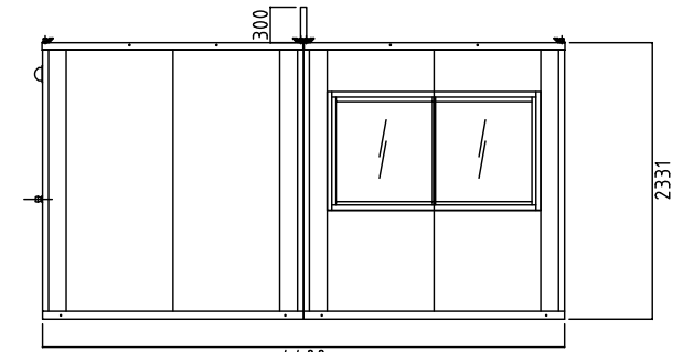
右側面図
