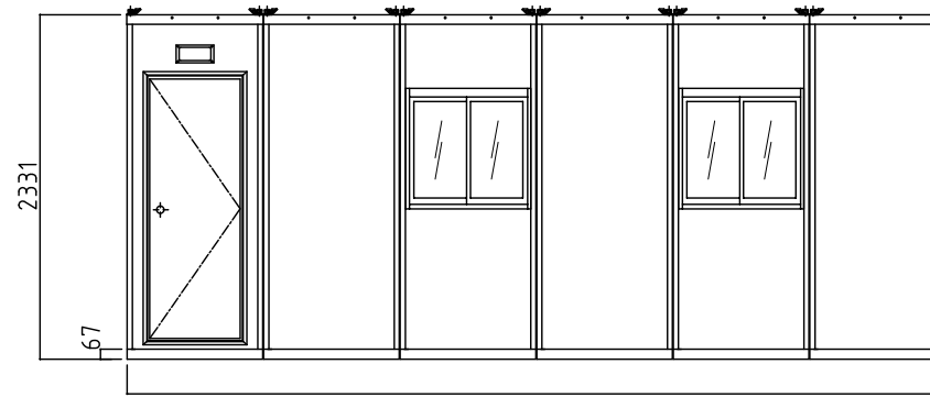
正面図
