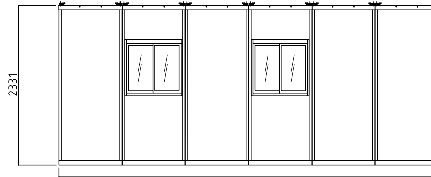
背面図
