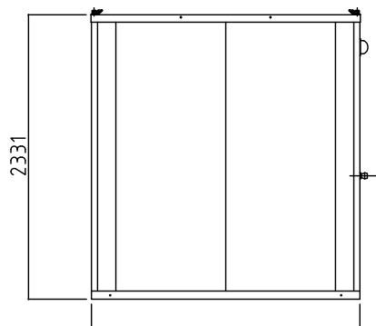
左側面図
