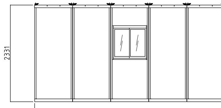
背面図
