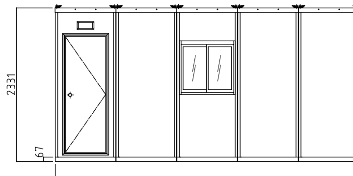
正面図
