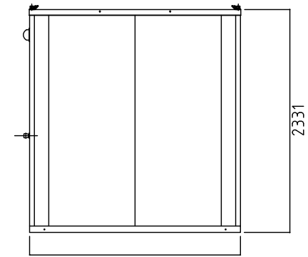
右側面図
