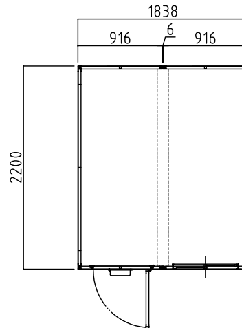
平面図
