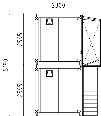
側面図
