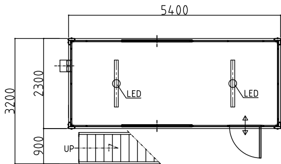
1F 平面図
