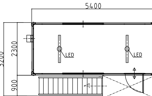
2F 平面図
