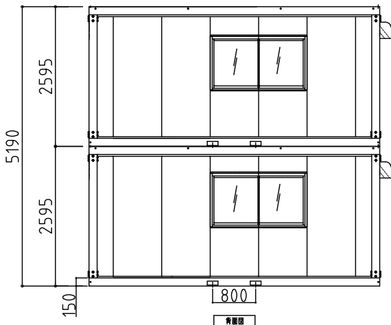
背面図
