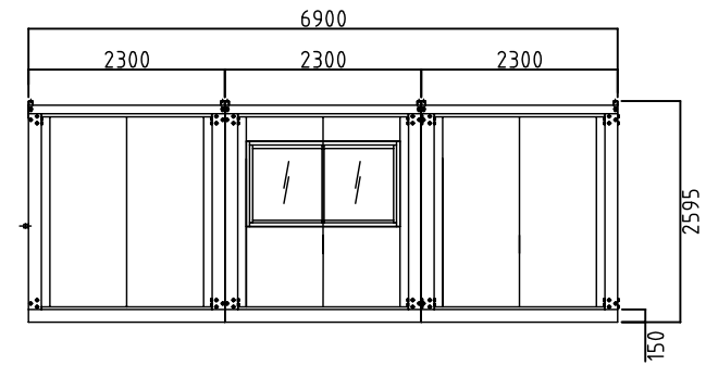
右側面図
