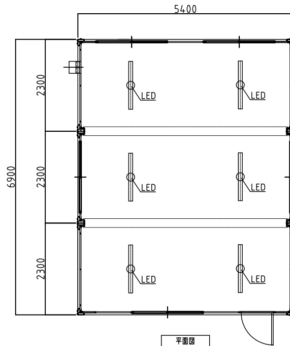
平面図
