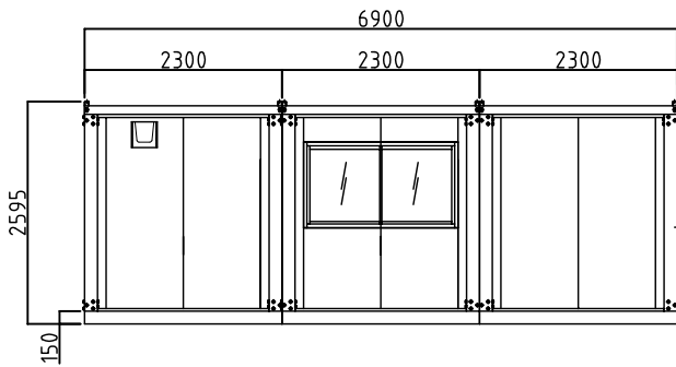
左側面図
