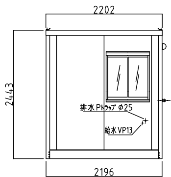
左側面図
