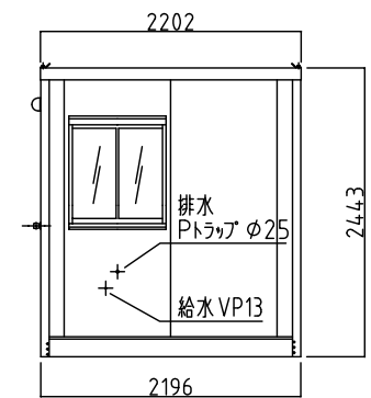
右断面図
