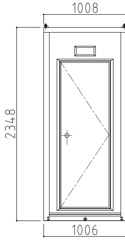
正面図
