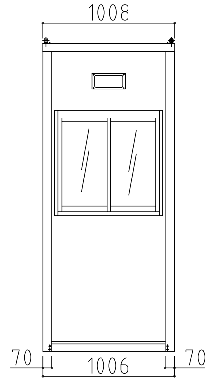
背面図
