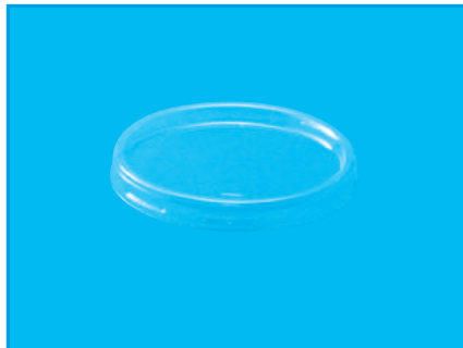
丸 60M オトシ蓋 21-702 ◆サイズ 66φ オトシ蓋 ◆ケース入数 5000枚 袋入数 100枚 ◆材質 A-PET ◆1枚重量 1g
