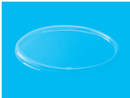
丸 MS-40-10 オートシ蓋 21-737 ◆サイズ 130φ共通 オートシ蓋 ◆ケース入数 1000枚 袋入数 50枚 ◆材質 A-PET ◆1枚重量 4.3g
