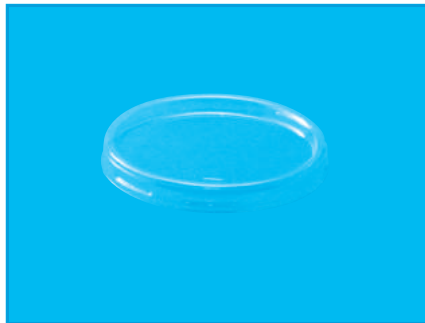
丸 60M オトシ蓋 21-702 ◆サイズ 66φ オトシ蓋 ◆ケース入数 5000枚 袋入数 100枚 ◆材質 A-PET ◆1枚重量 1g
