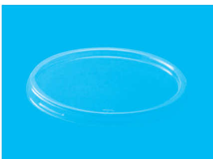
丸 MS-20 オトシ蓋 21-713 ◆サイズ 100φ共通 オトシ蓋 ◆ケース入数 2500枚 袋入数 100枚 ◆材質 A-PET ◆1枚重量 2.4g
