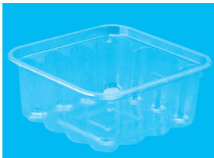
角菊 KG-470B 21-624 ◆サイズ 125×125×52mm ◆ケース入数 1500枚 袋入数 100枚 ◆材質 A-PET ◆1枚重量 10.7g
