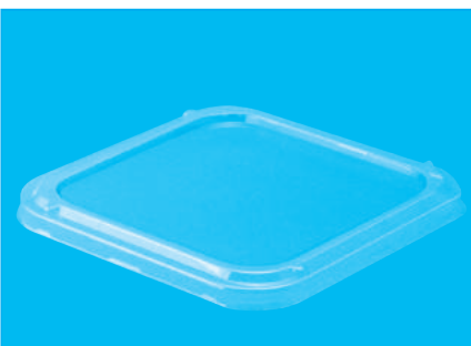
角 GK カブセ蓋 21-626 ◆サイズ 125角共通 カブセ蓋 ◆ケース入数 1500枚 袋入数 100枚 ◆材質 A-PET ◆1枚重量 4.9g
